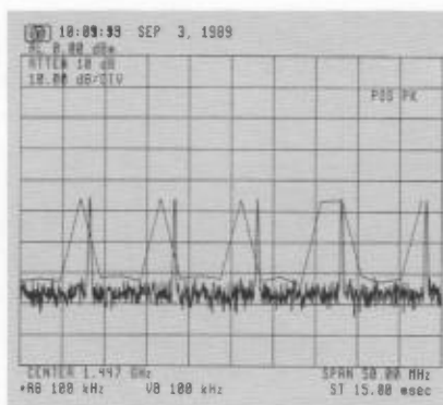
Fig. 35. Pos peak display mode versus actual comb.
