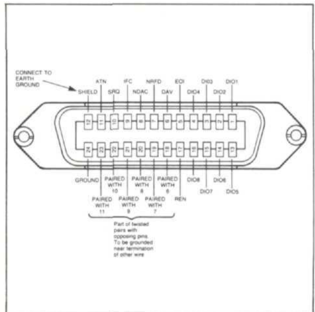
IEEE/ANSI connector
